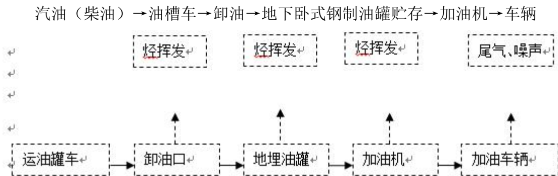
图 2 站场营运期加油工艺流程及产污环节图
