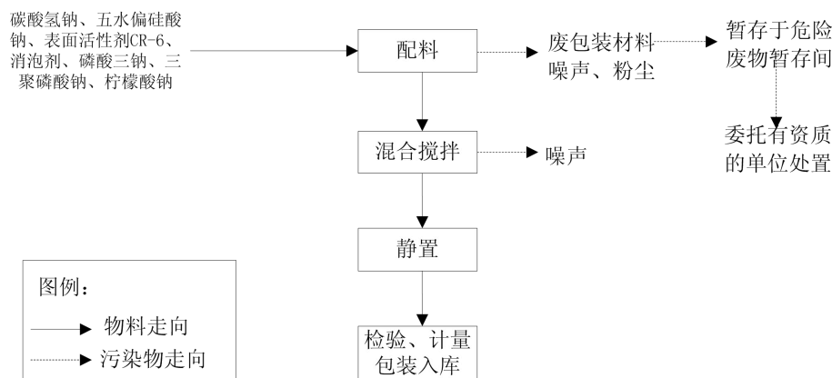
图 2.1-4 脱脂剂生产工艺流程及产污环节
