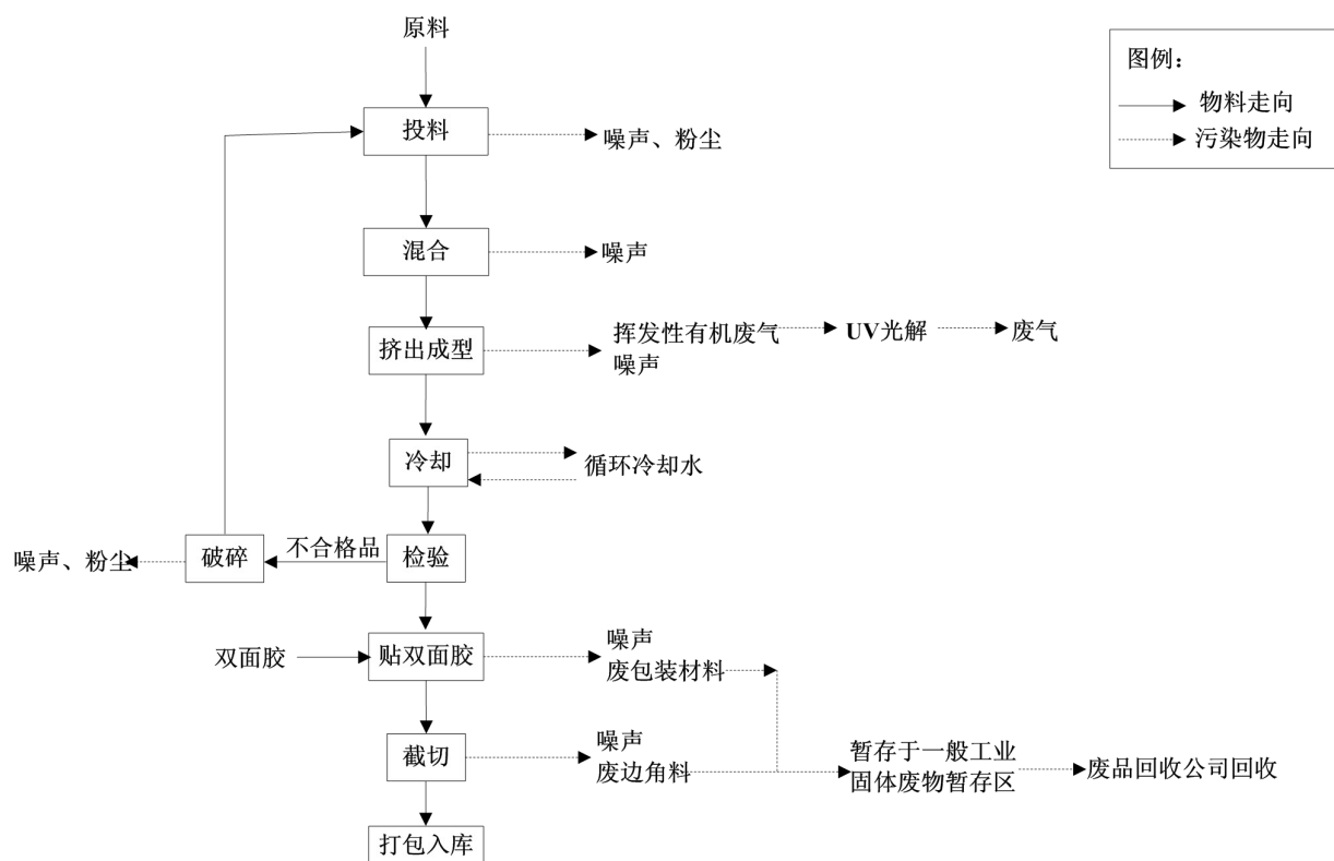
图 2.1-5 PVC 防火胶条生产工艺流程及产污环节
