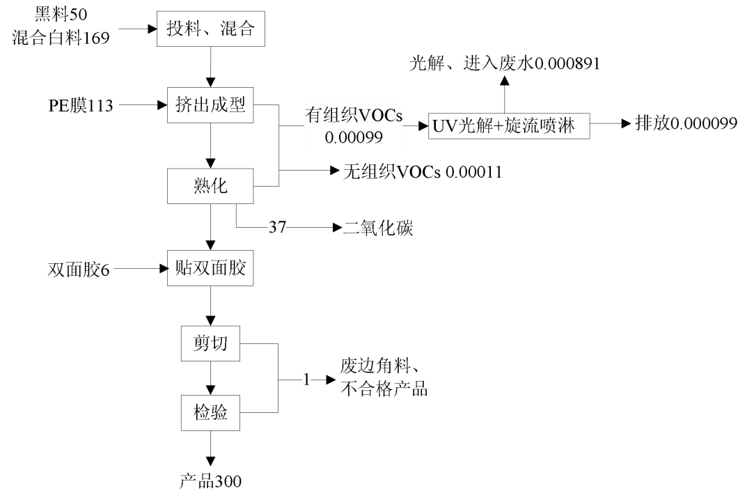
图 3.2-5 普通胶条生产线物料平衡图 t/a
