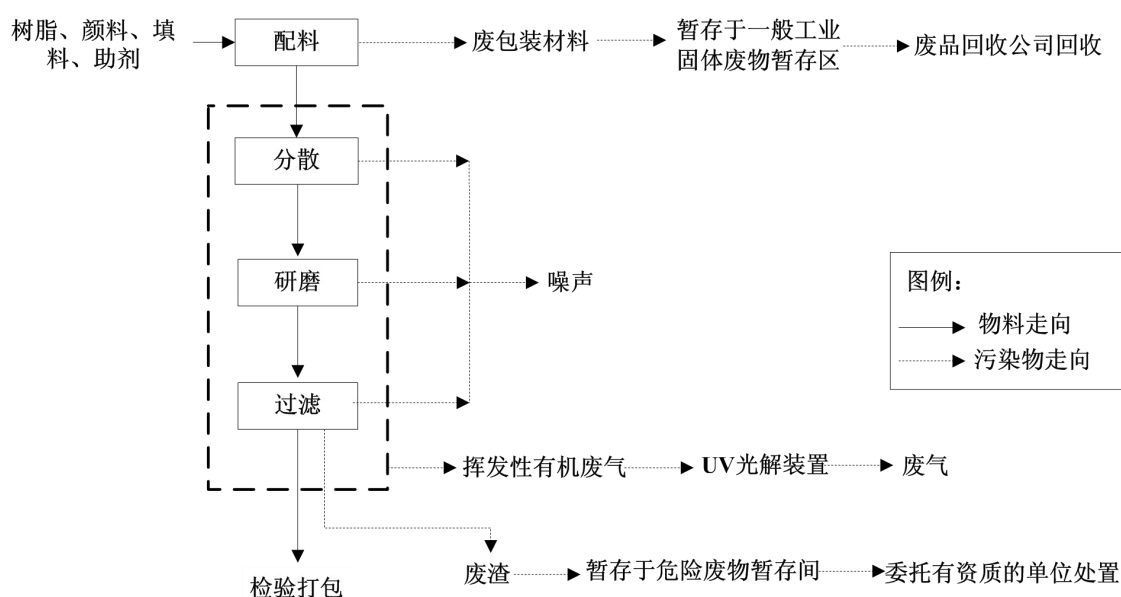
图 2.1-1 油性漆生产工艺流程及产污环节
