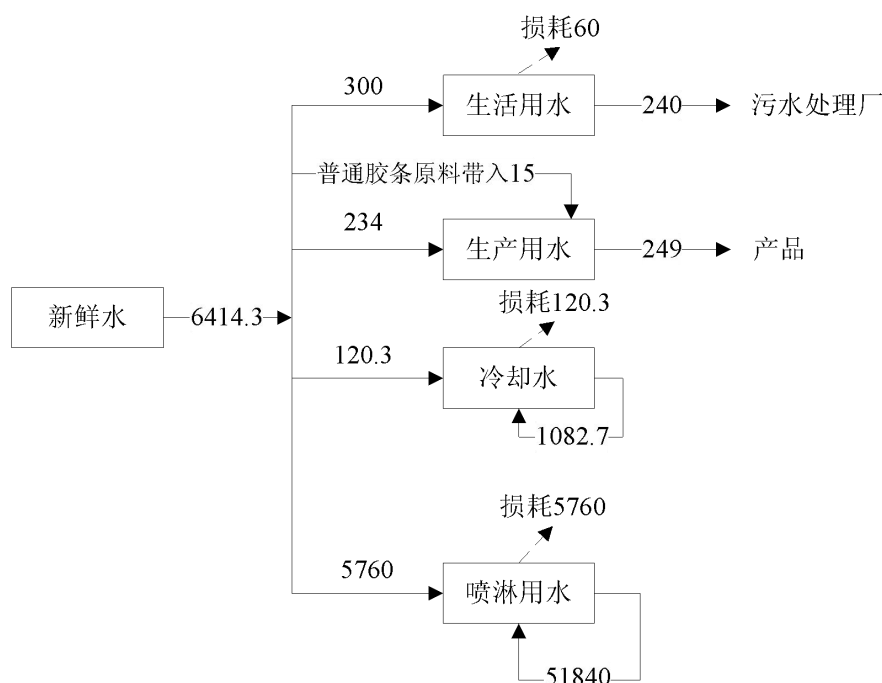
图 3.2-7 本次扩建水平衡图 单位： \text{m}^3/\text{a}
