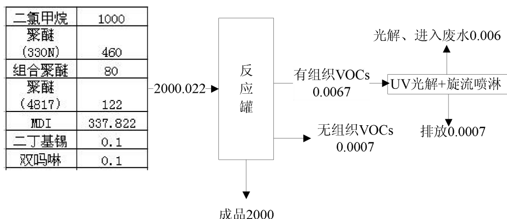
图 3.2-6 发泡胶生产线物料平衡图 t/a
