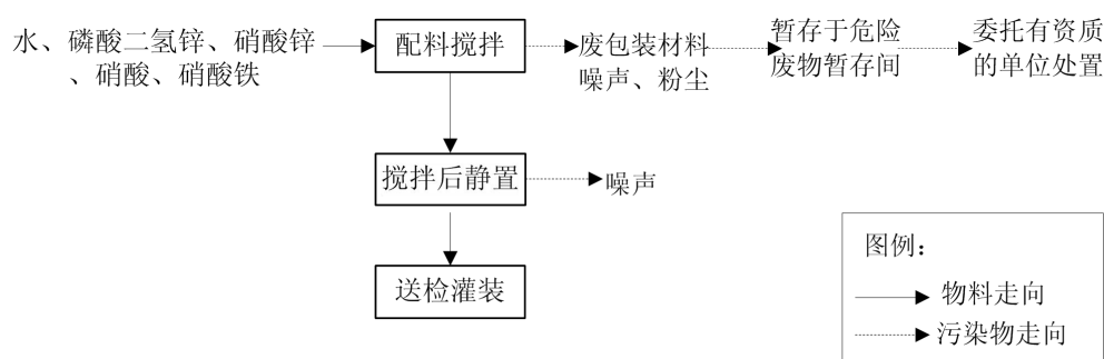
图 2.1-3 磷化液生产工艺流程及产污环节
