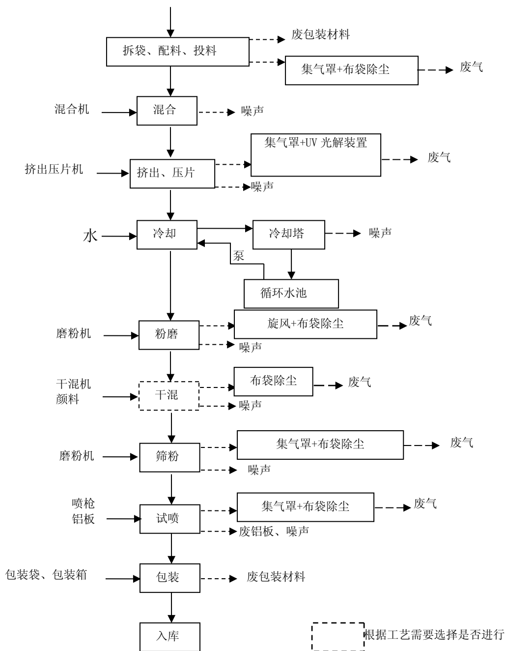
图 2.1-2 环氧树脂粉末生产工艺流程及产污环节
