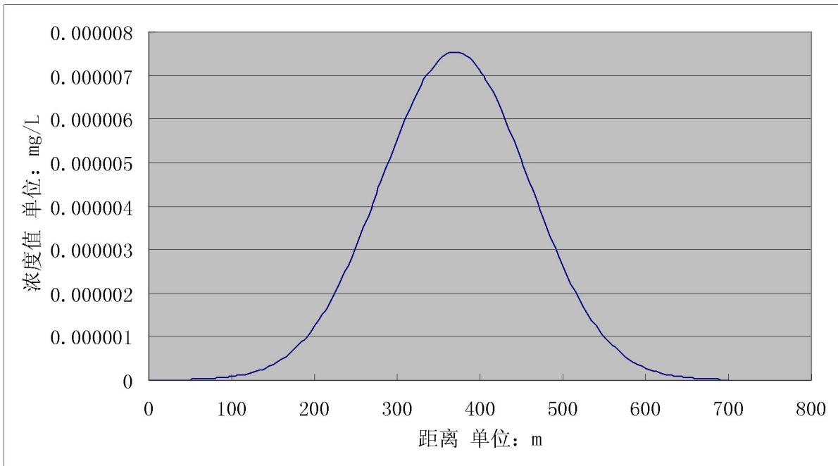
图 5.2-2 泄漏第 1000 天，二氯甲烷污染扩散距离图
