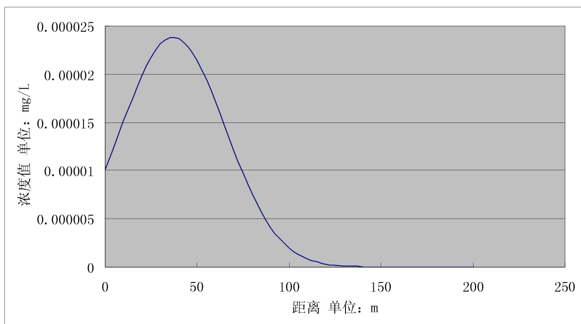
图 5.2-1 泄漏第 100 天，二氯甲烷污染扩散距离图
