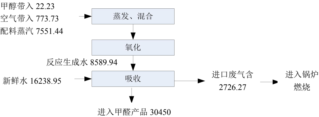
图 3.2-2 甲醛生产线水平衡图（单位：m³/a）
