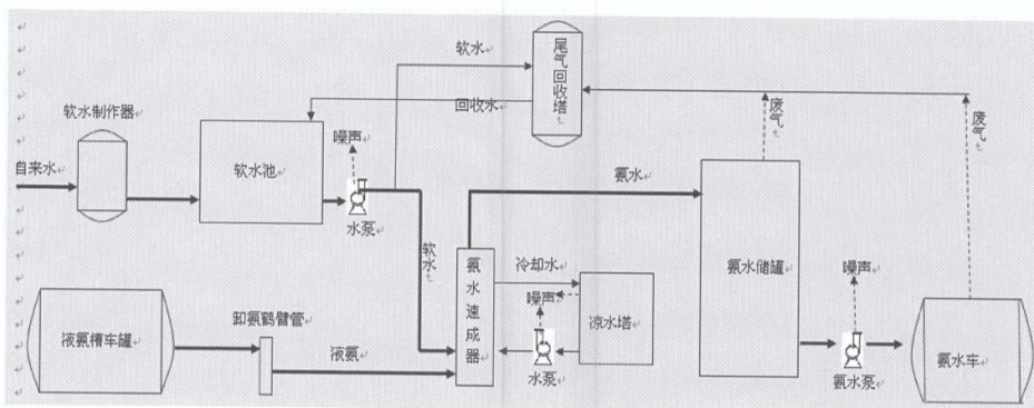
图 1 年产 6 万吨氨水项目运营期生产工艺及产污流程图
