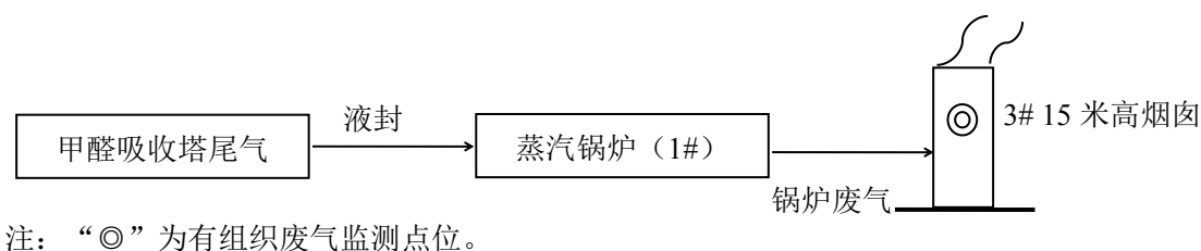
图 4-1 废气治理工艺流程图
