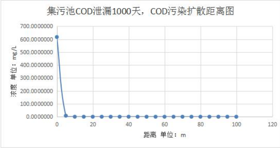
图4.2.3-2 集污池COD泄漏1000天，COD污染扩散距离图
