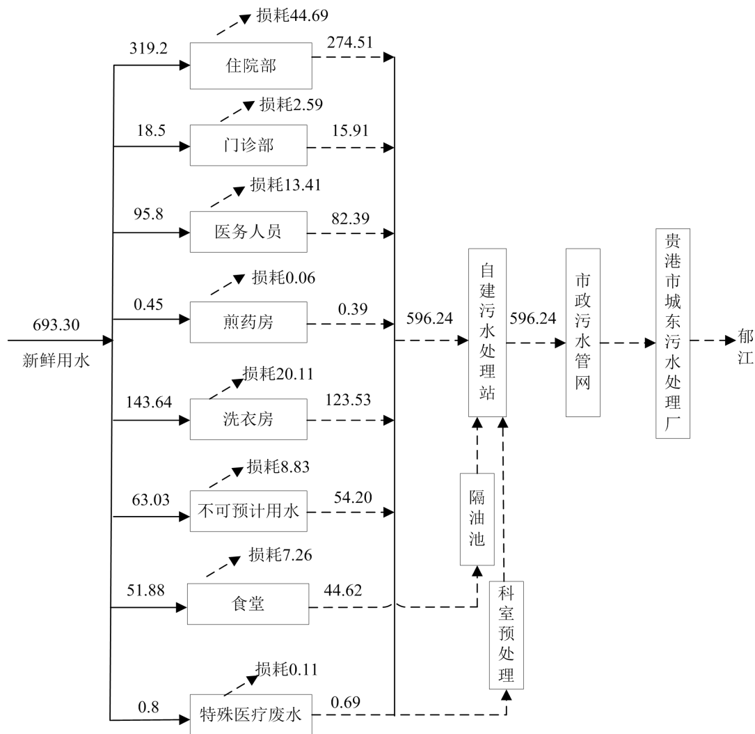
图3.3-1 项目运营期水平衡示意图 (单位: m³/d)
