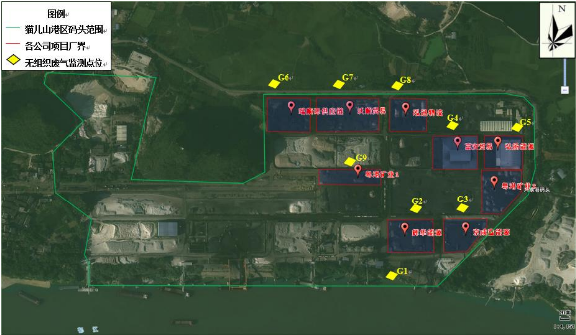
图 3-1 无组织废气监测点位示意图
