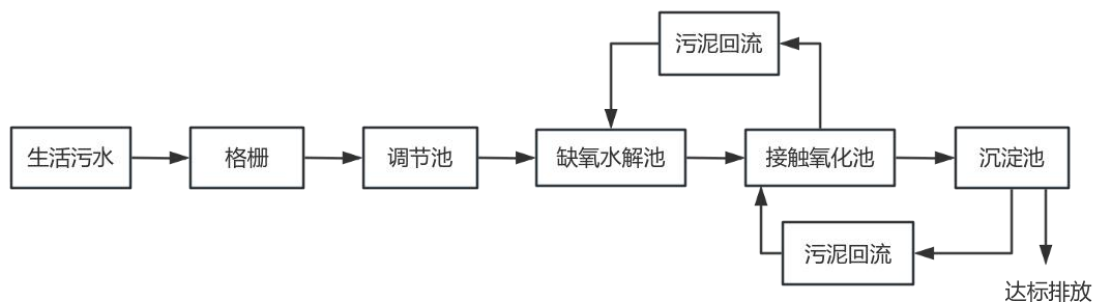
图 3-4 生活污水处理站（依托）工艺流程图
