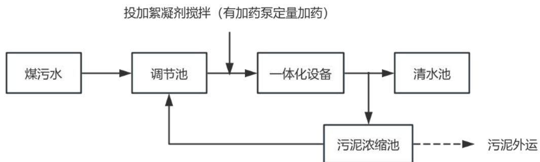
图 3-3 煤污水处理站（依托）工艺流程图
