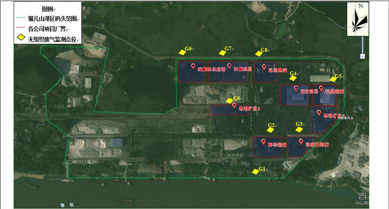
图 3-1 无组织废气监测点位示意图
