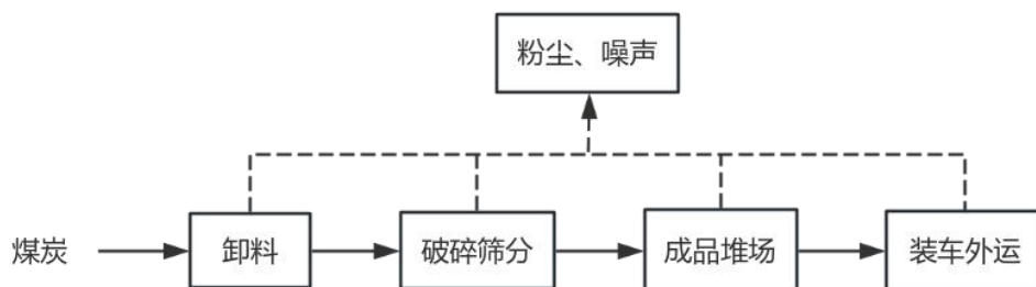
图 2-1 生产工艺流程及产污节点图
